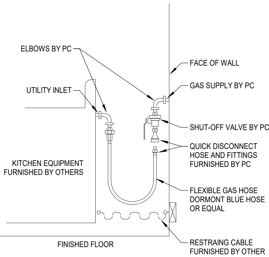
6 GAS QUICK CONNECT DETAIL Scale: N.T.S.
