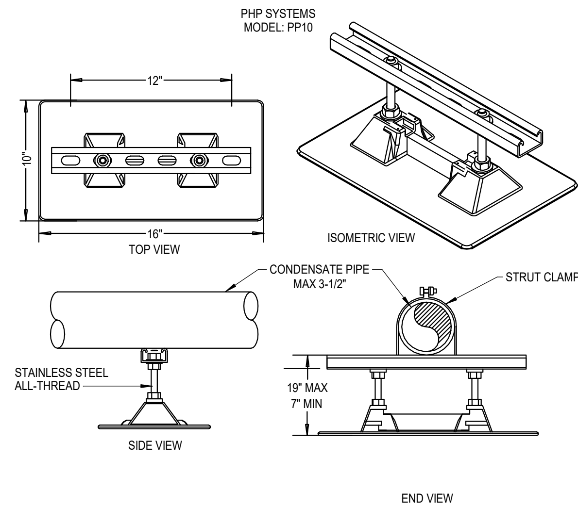
6 CONDENSATE PIPE SUPPORT ON ROOF Scale: N.T.S.
