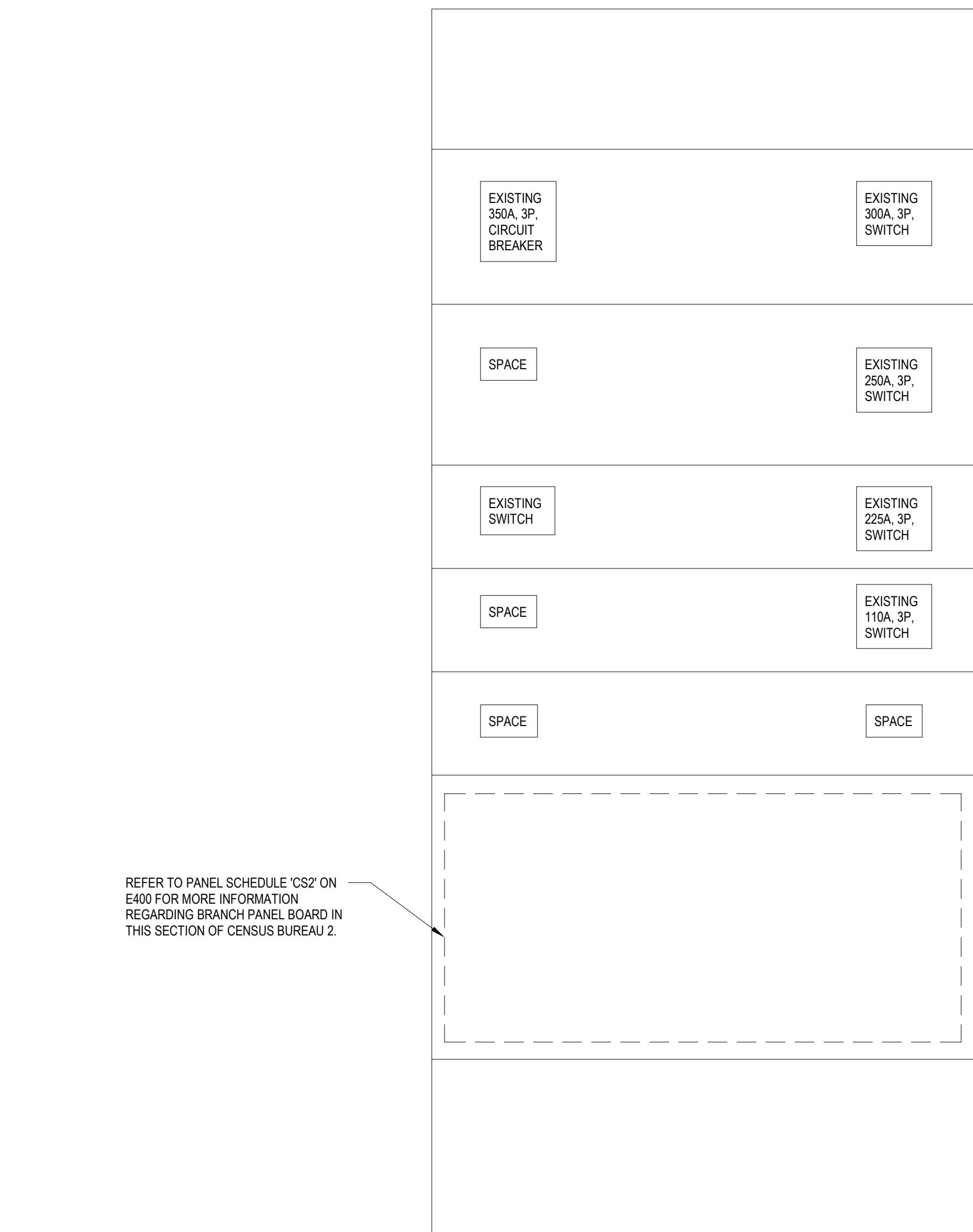
3 CENSUS BUREAU 2 SWITCHBOARD DESIGN E300 SCALE: N.T.S.
