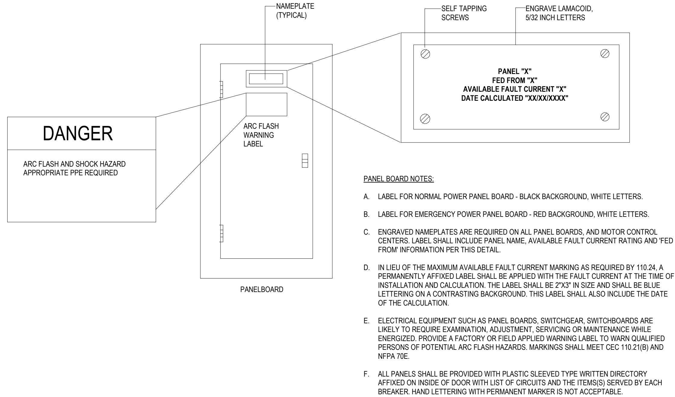
2 PANEL LABEL DETAIL E300 SCALE: N.T.S.
