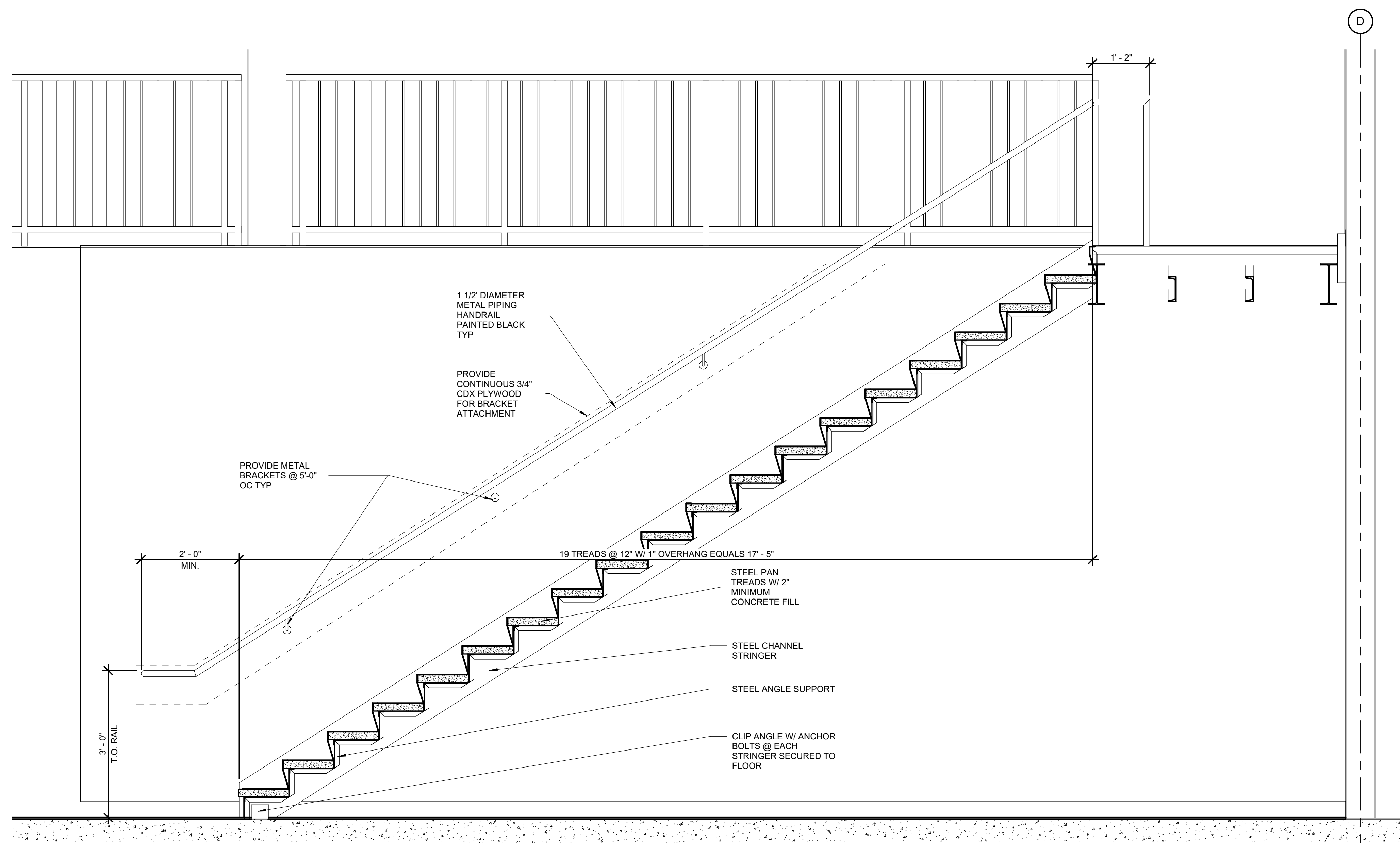
11 STAIR SECTION SCALE: 3/4" = 1'-0"
