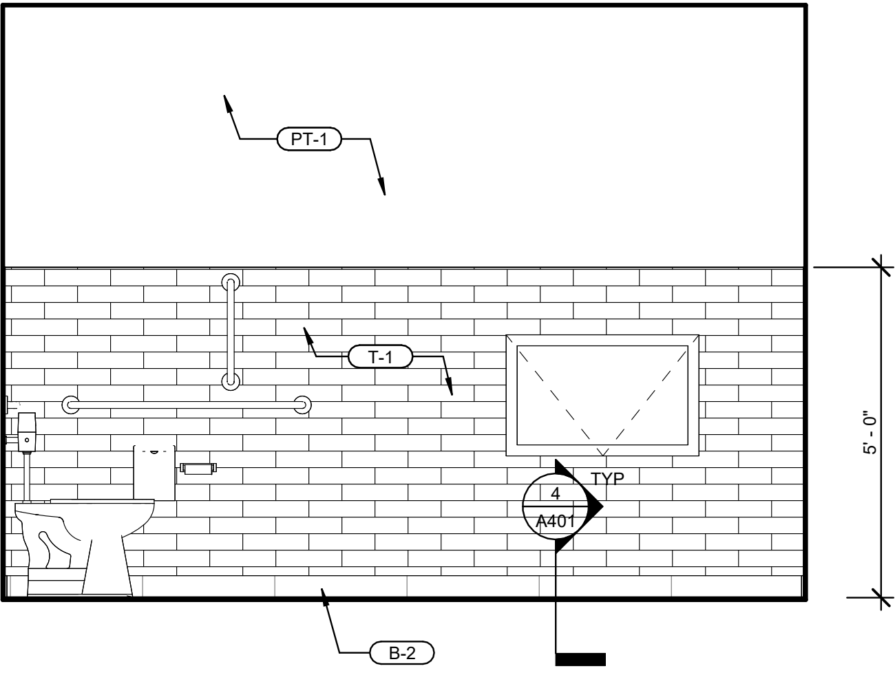
② WOMEN SCALE: 1/2" = 1'-0"
