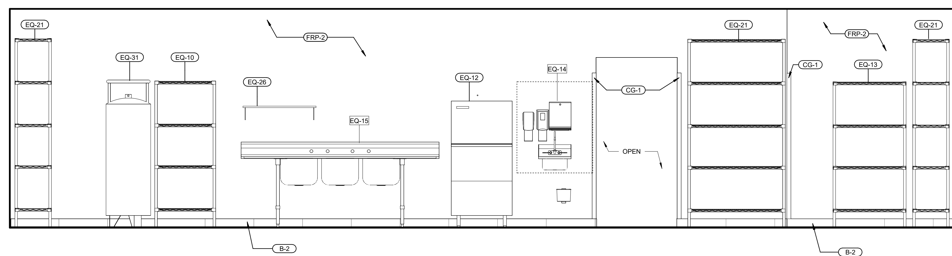
① PREP AREA SCALE: 1/2" = 1'-0"
