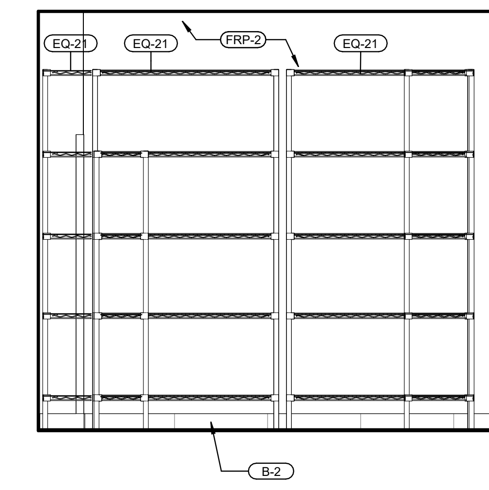
④ PREP AREA SCALE: 1/2" = 1'-0"
