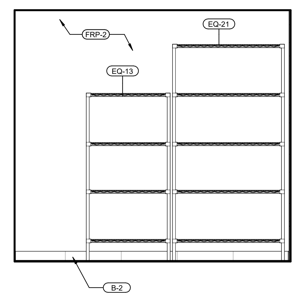
② PREP AREA SCALE: 1/2" = 1'-0"
