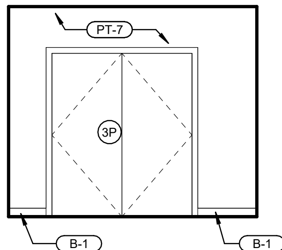
3 CORRIDOR SCALE: 1/4" = 1'-0"
