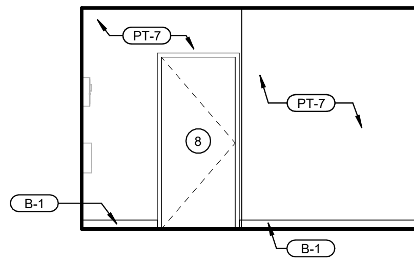
7 STORAGE SCALE: 1/4" = 1'-0"
