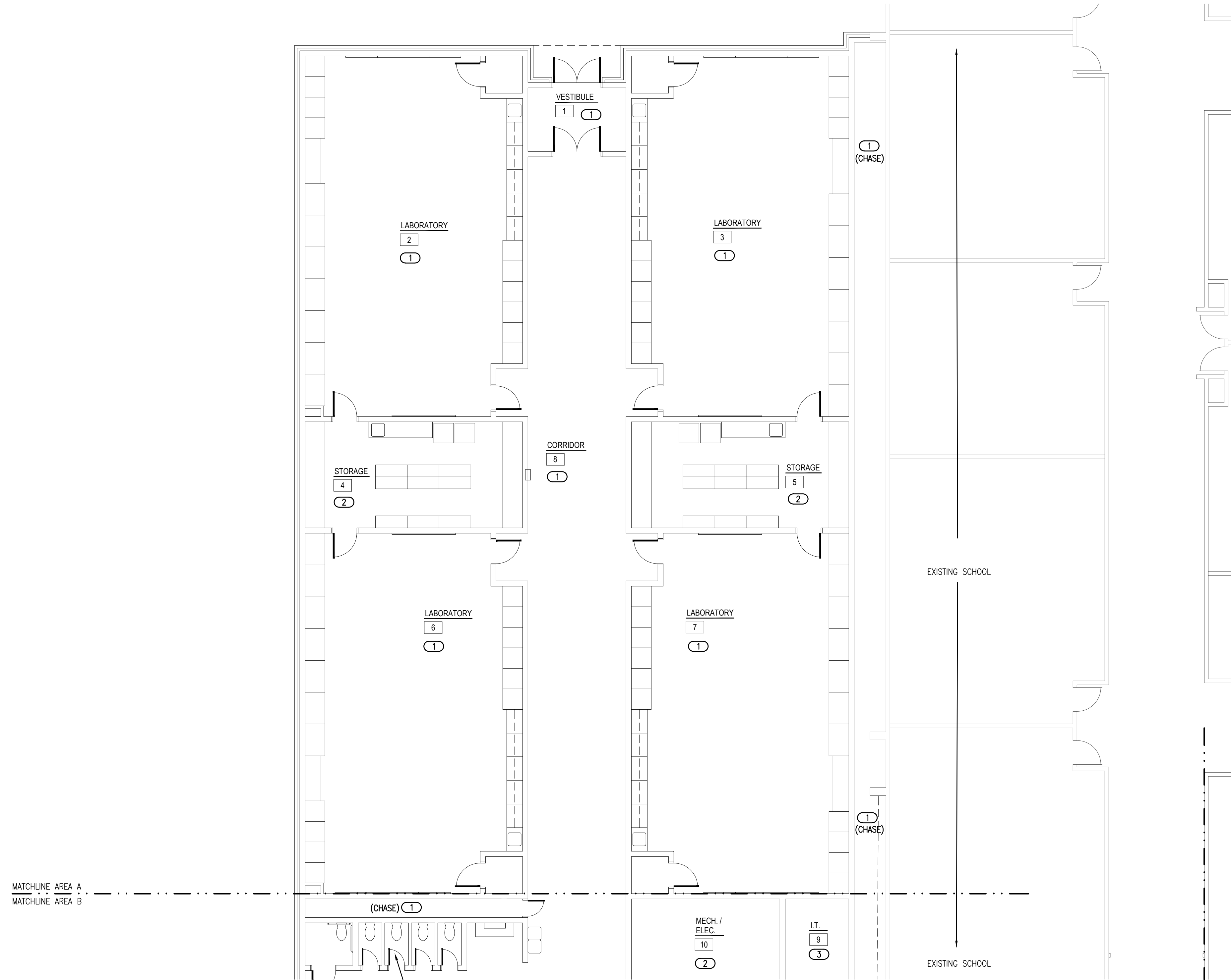
1 FIRE PROTECTION PLAN - AREA A SCALE: 1/8" = 1'-0"
